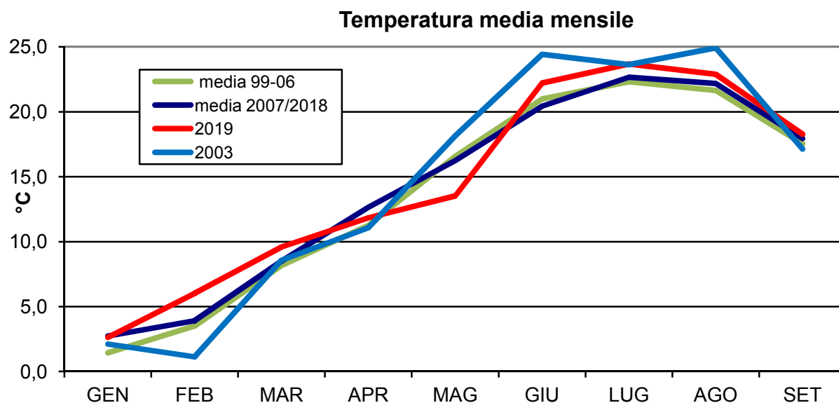
Grafico 5 – temperature medie mensili, stazione della Regione Piemonte, Sesto (NO)
