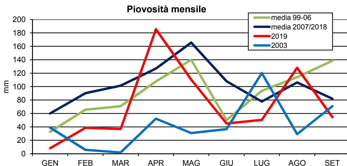
Grafico 6 –pioggia cumulata mensile, stazione della Regione Piemonte, Sesto (NO).
